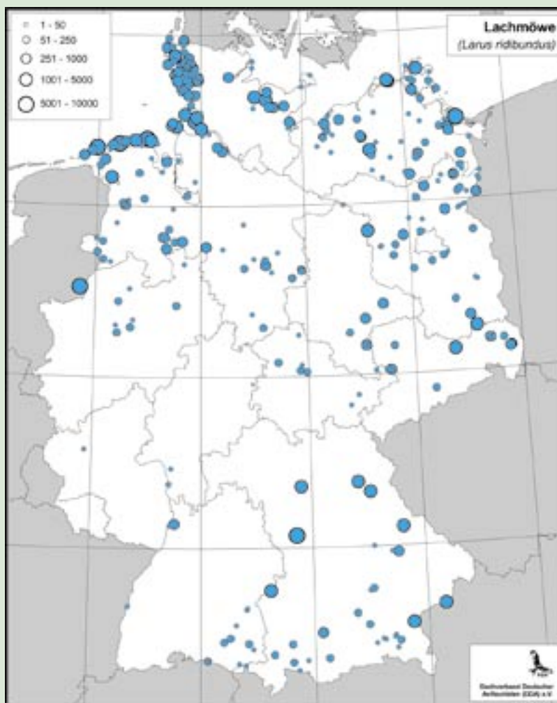
Verbreitung der Lachmöwe in Deutschland 1999.
